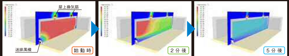
送風機
