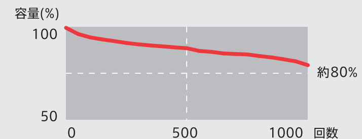
充放電サイクル特性（当社試験結果による）
