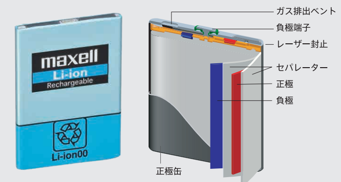
マクセル製 角形リチウムイオン電池
